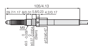
DK812AFR/DK812AFR5 DK812BFR/DK812BFR5
