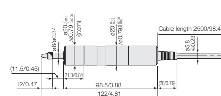
DK10NR5/PR5
