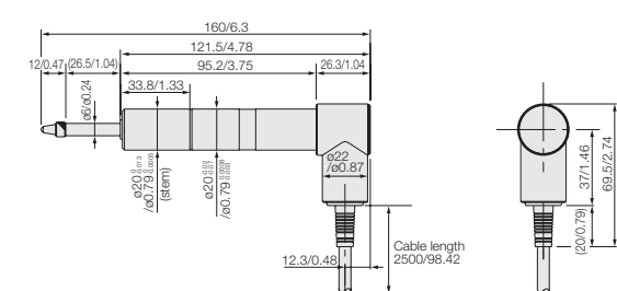
DK25NLR5/PLR5
