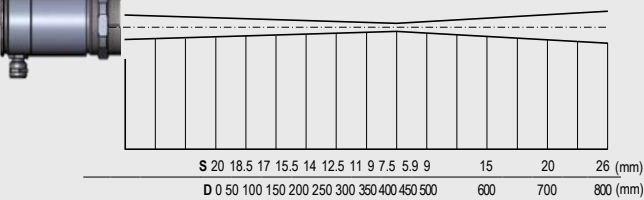
CF4 optics 75:1
