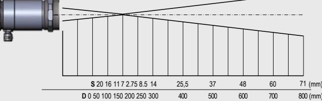
CF3 optics 75:1
