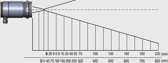
CF3 optics 75:1
