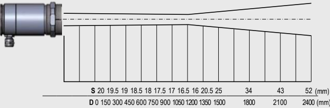
CF2 optics 75:1
