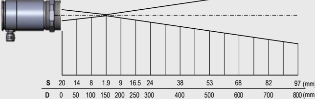
CF2 optics 75:1
