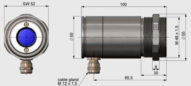
센서 헤드
